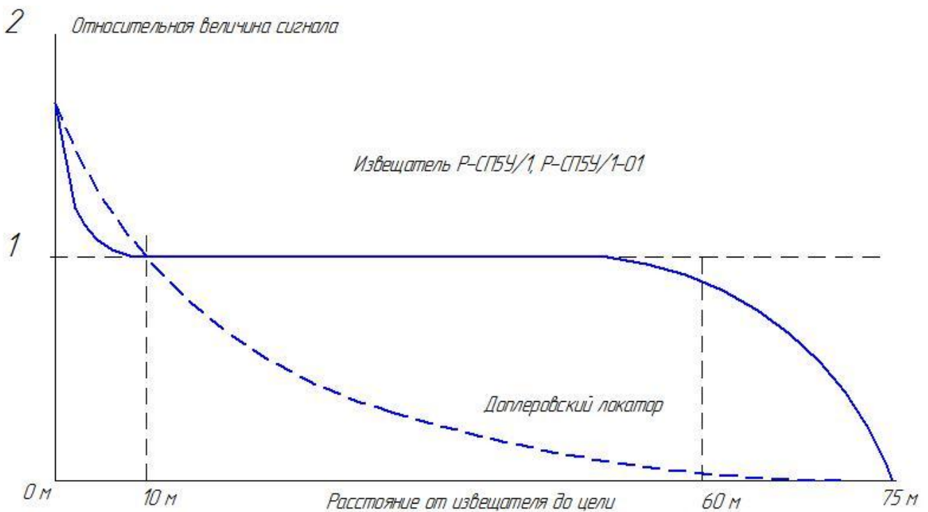
Рисунок 1.4 – Зависимость сигнала Р-СП5У/1, Р-СП5У/1-01 от расстояния
