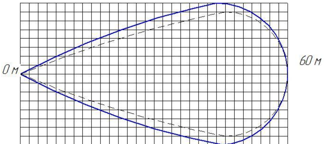
Рисунок 1.2 – Примерная форма ЗО Р-СП5У/1, Р-СП5У/1-01 при максимальной дальности
