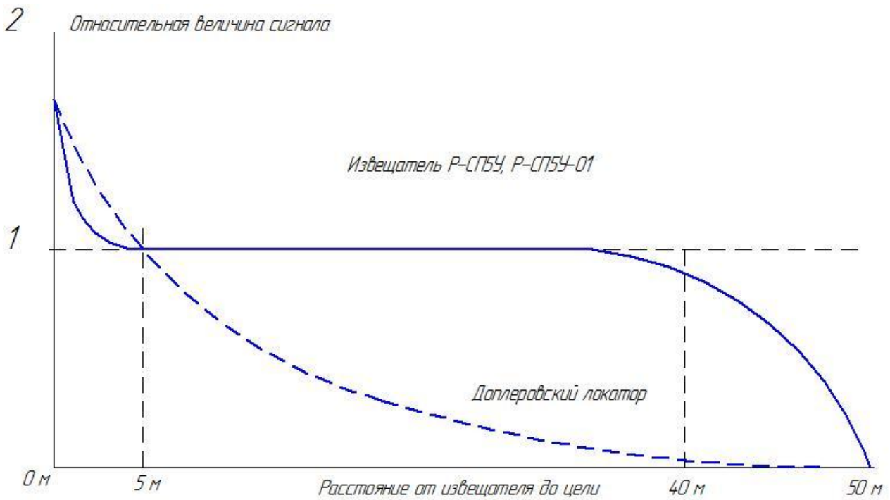
Рисунок 1.3 – Зависимость сигнала Р-СП5У, Р-СП5У-01 от расстояния
