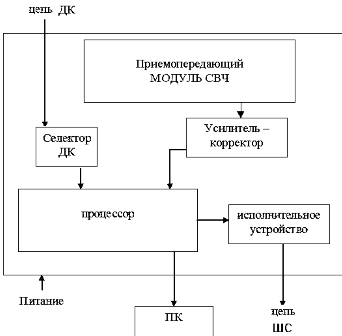
Рисунок 1.5 – Упрощенная функциональная схема
