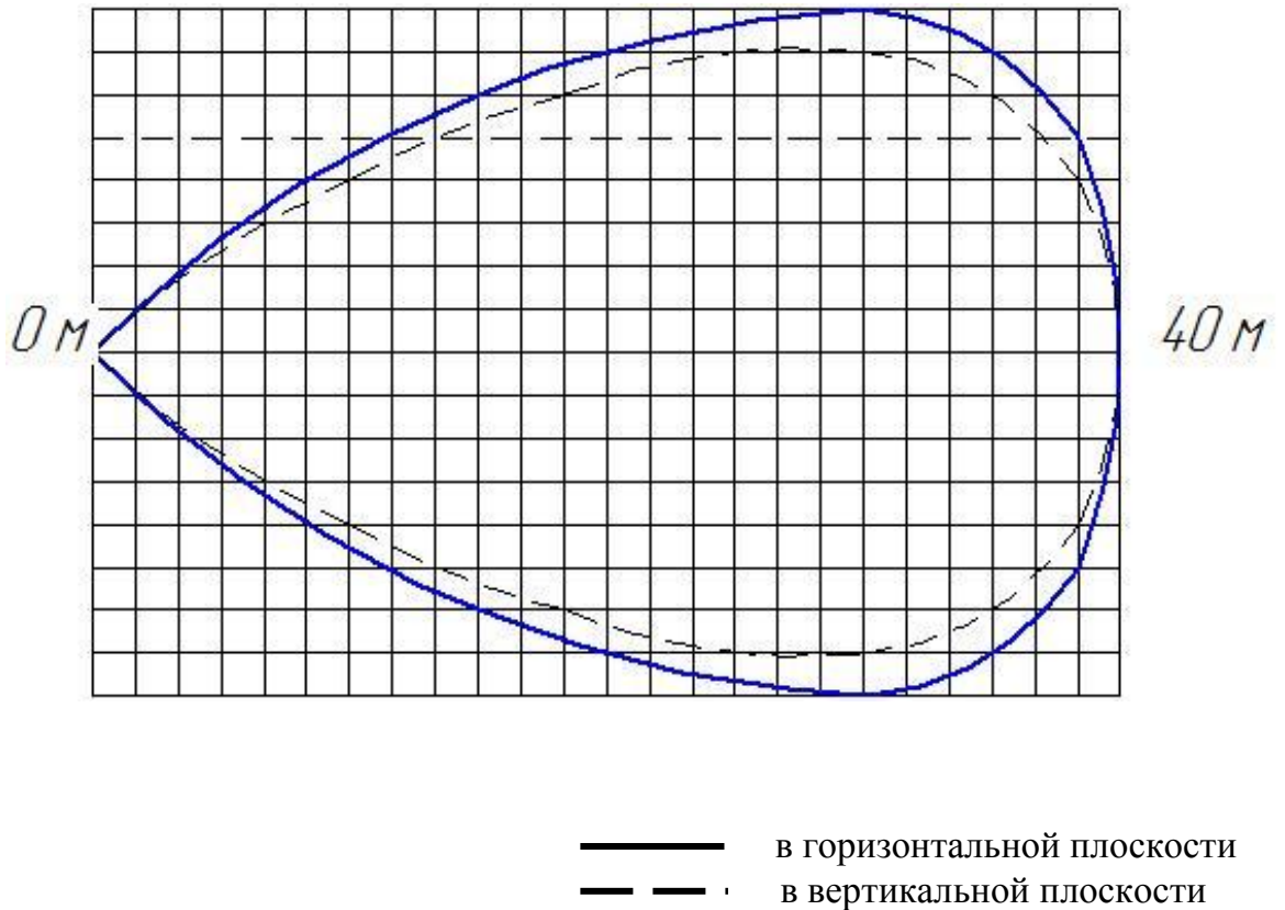
Рисунок 1.1 – Примерная форма ЗО Р-СП5У, Р-СП5У-01 при максимальной дальности
