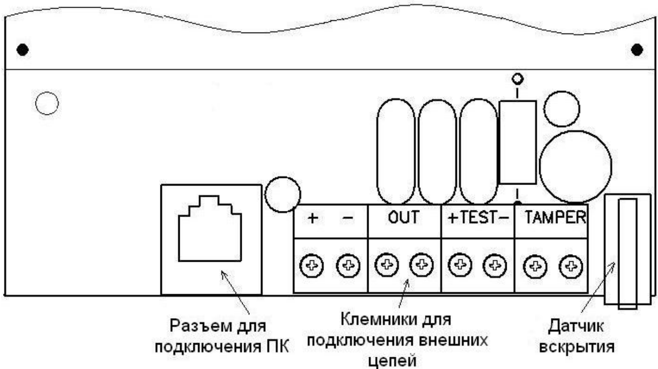
Рисунок 1.7 – Органы коммутации ПРМ-ПРД извещателей Р-СП5У-01 и Р-СП5У/1-01
