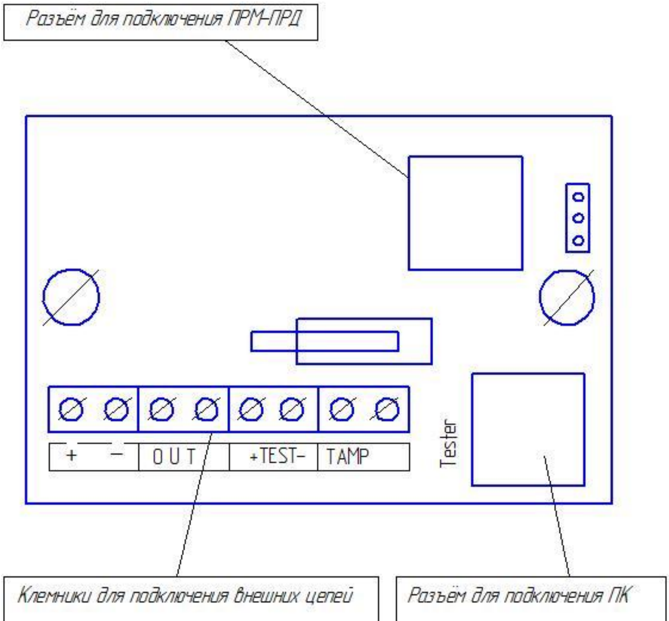
Рисунок 1.6 – Органы коммутации КР
